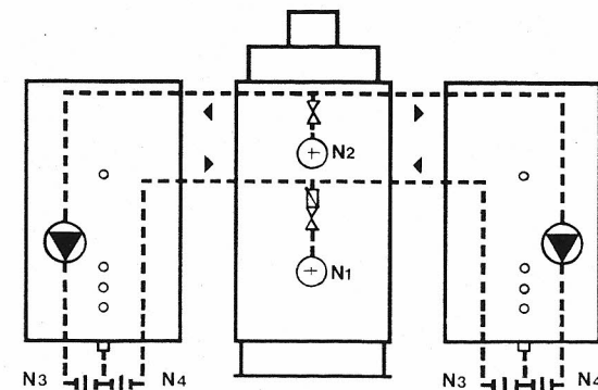
D: caldaia con 2 boiler laterali
